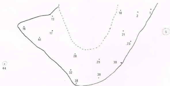
FIG. 5. — Aréologie de \frac{40}{\text{« S »}} (ALMC 20).
