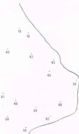
FIG. 4. — Aréologie de \frac{4}{\text{« S »}} ( ALMC 20).
