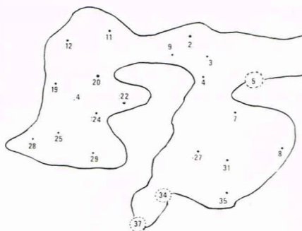
FIG. 6. — Aérologie de \frac{1}{S} (ALMC 20)
