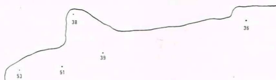
FIG. 3. — Aréologie de \frac{3}{\text{«S»}} ( ALMC 20).
