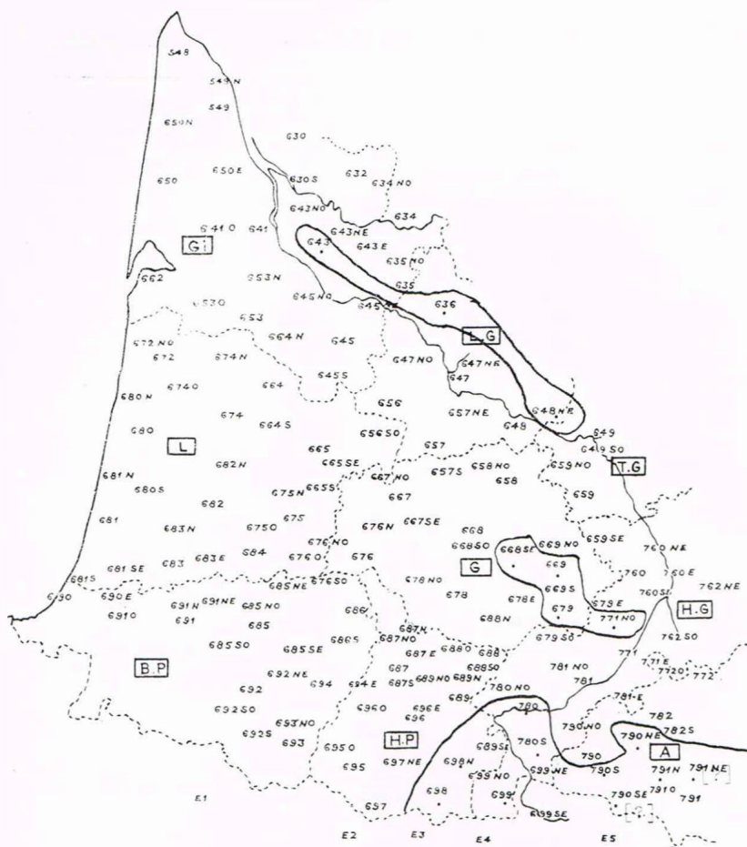
FIG. 7 bis.— Aire des unités ponctuelles à distance zéro; le signifiant Altan signifie « vent du sud ».
